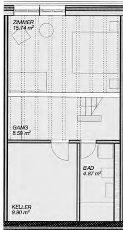
B-2 1. Untergeschoss
