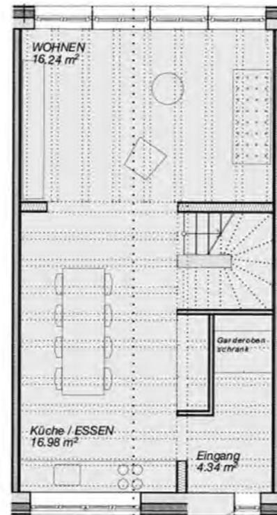
B-2 Erdgeschoss
