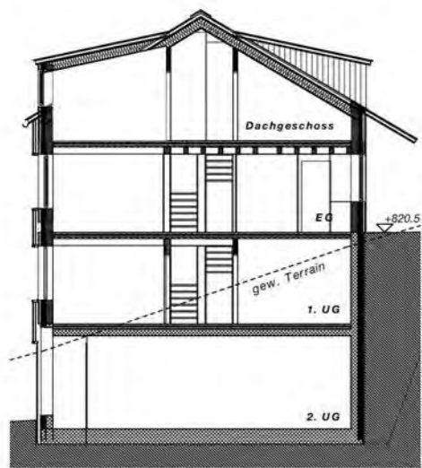
Schnitt Haus B MST 1:200
