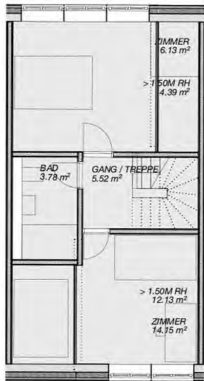
B-2 Dachgeschoss
