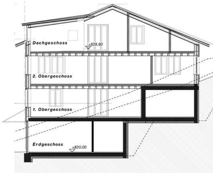
Schnitt Haus A MST 1:200
